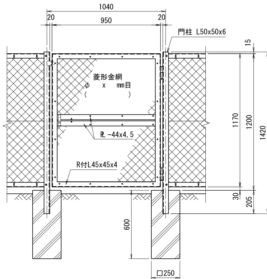
正面図 (S=1/20)
