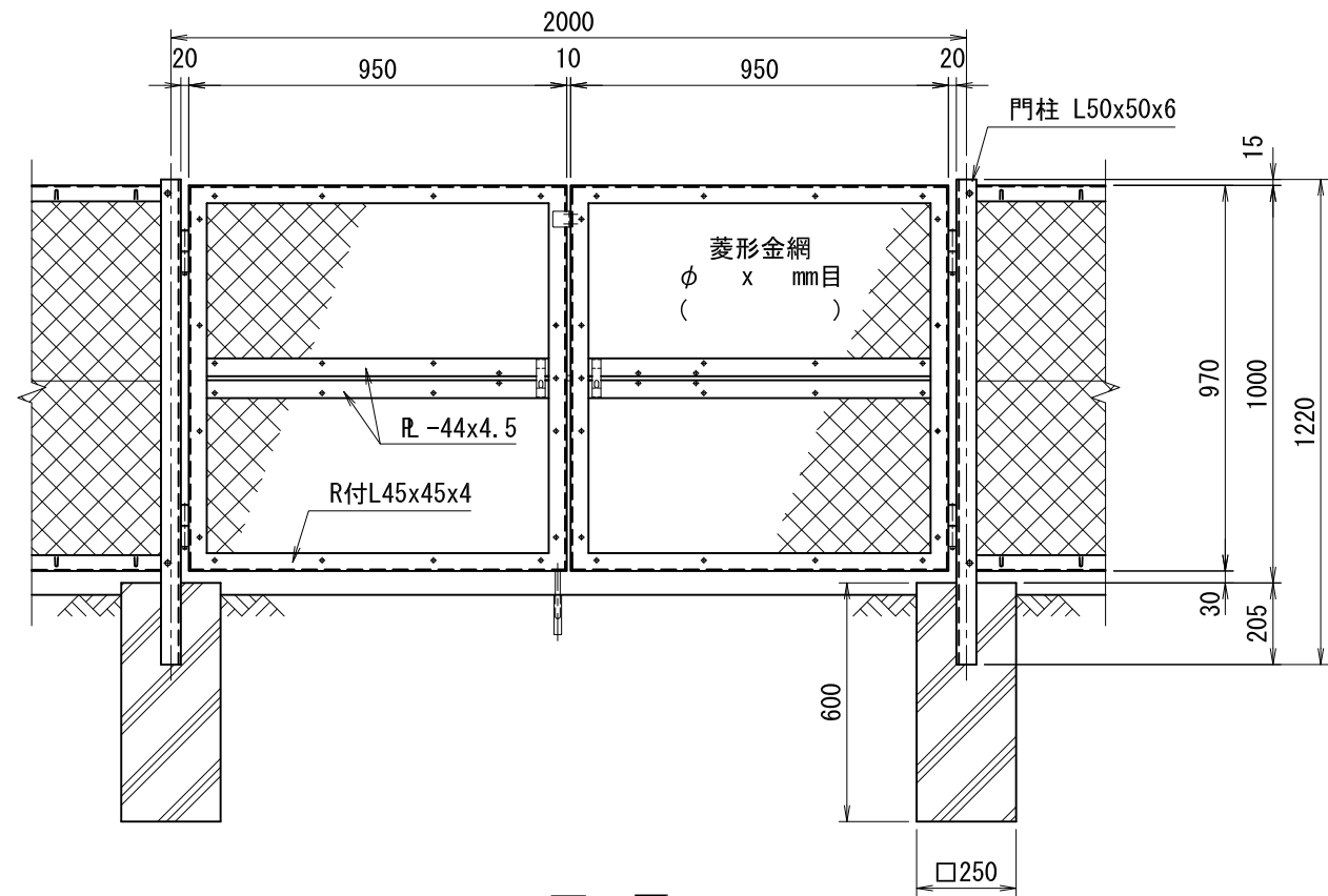
正面図 (S=1/20)
