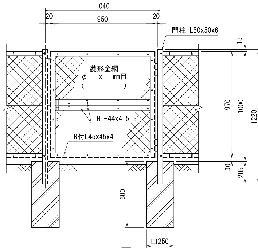
正面図 (S=1/20)
