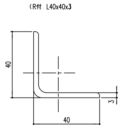
胴縁断面図 S=1/1
