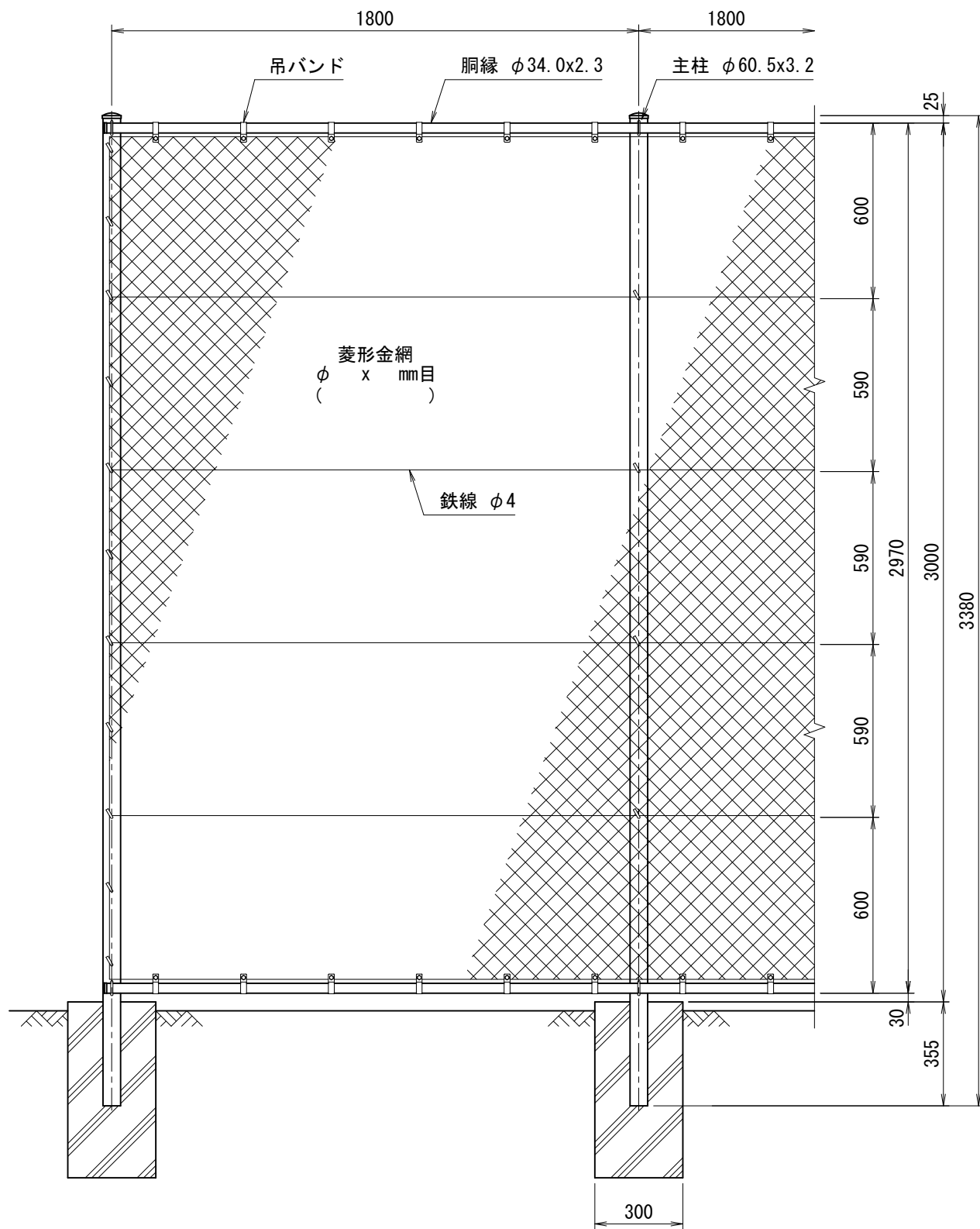
正面図 (S=1/20)
