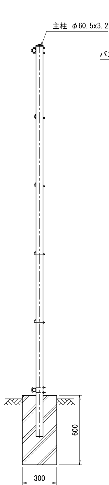
側面図 (S=1/20)
