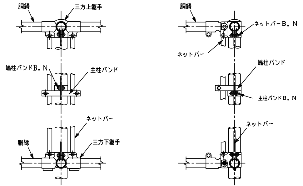
三方部取付詳細
