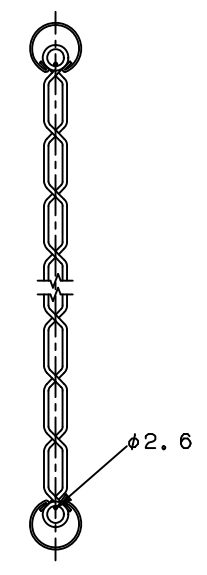
胴縁と金網取付断面図
