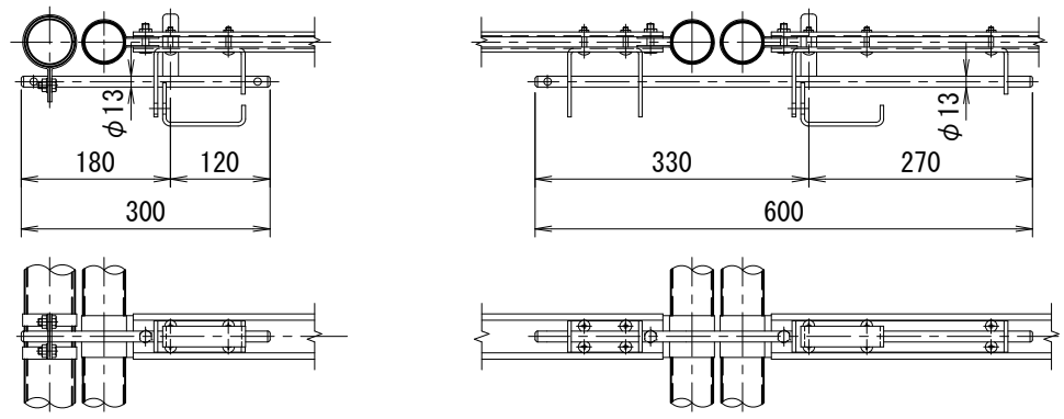
カンヌキ取付詳細図
