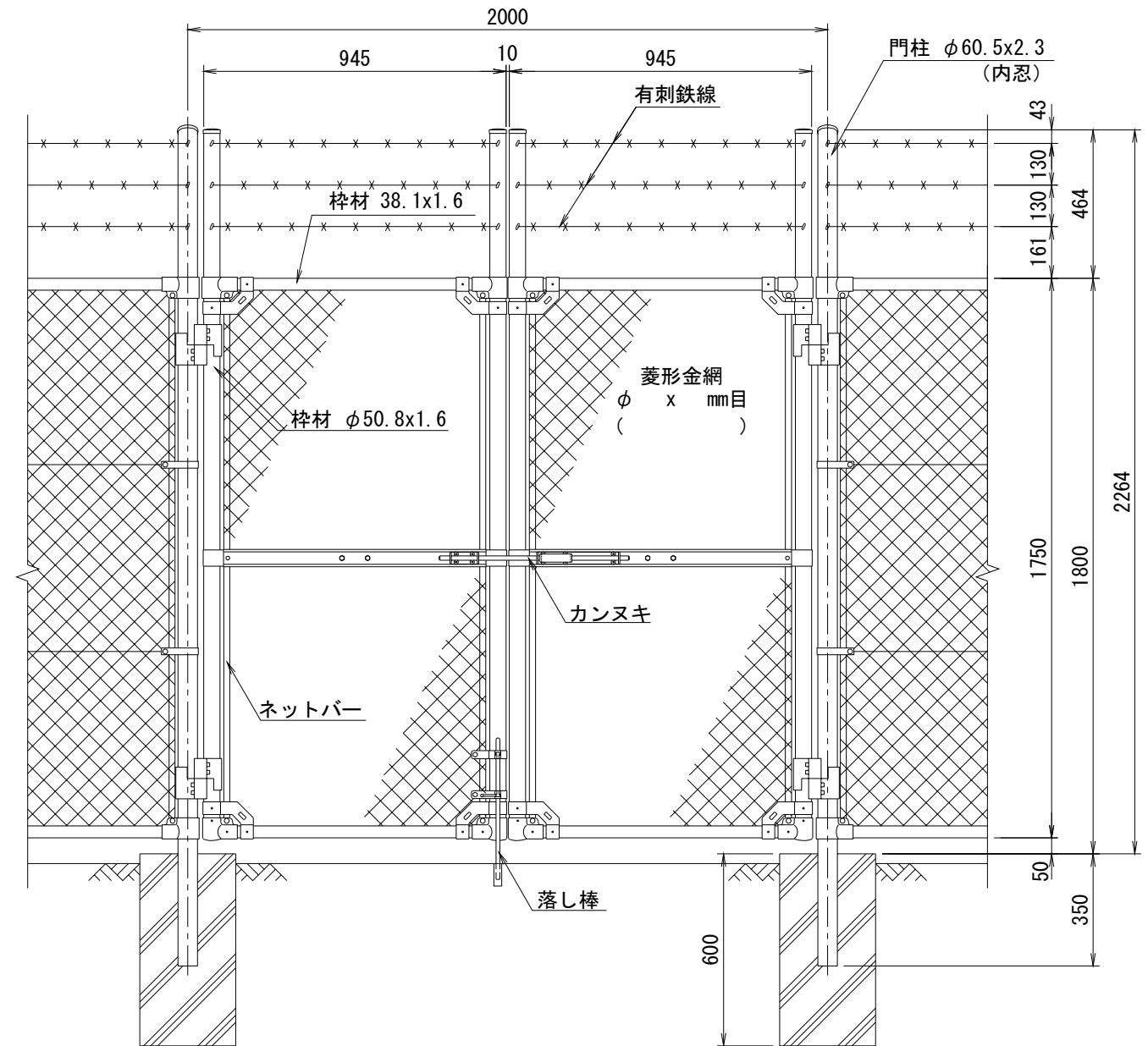
正面図 (S=1/20)
