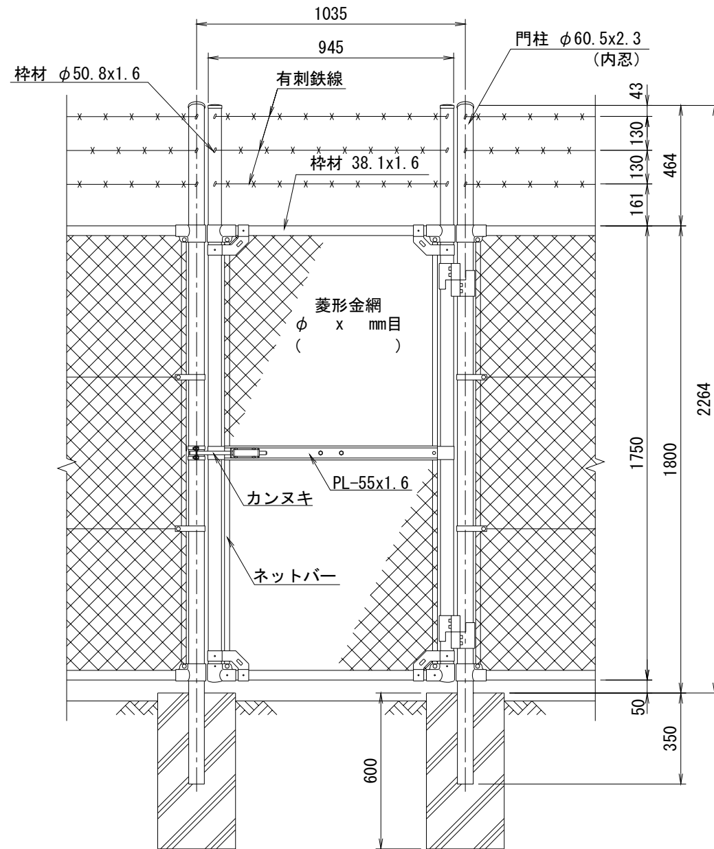
正面図 (S=1/20)
