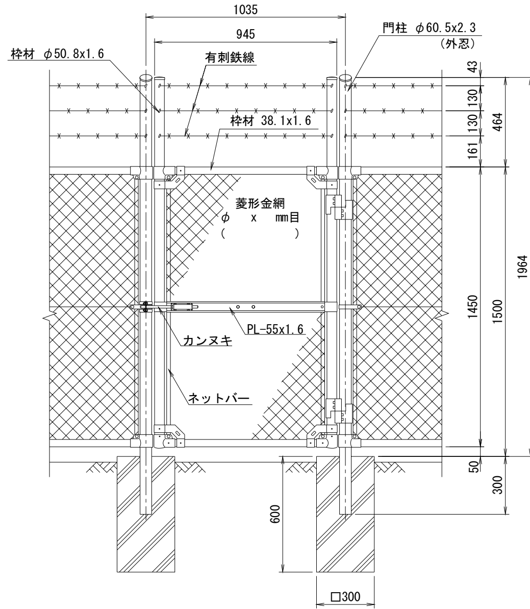
正面図 (S=1/20)
