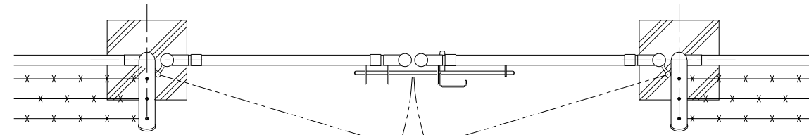
平面図 (S=1/20)
