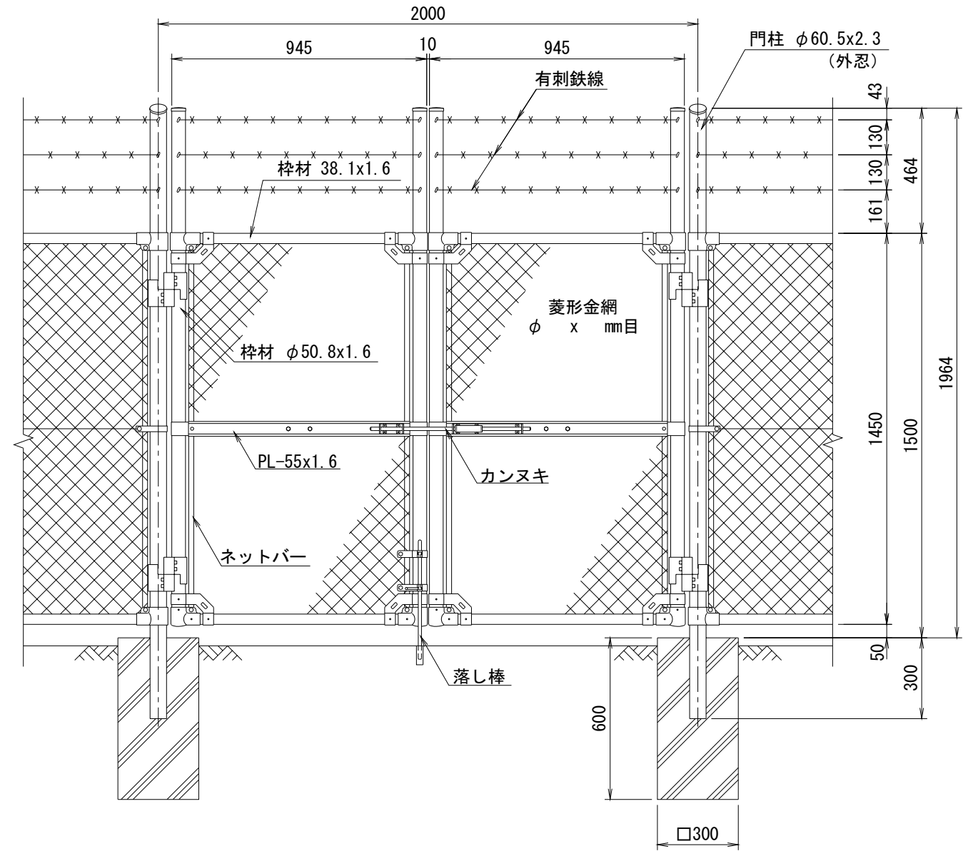
正面図 (S=1/20)
