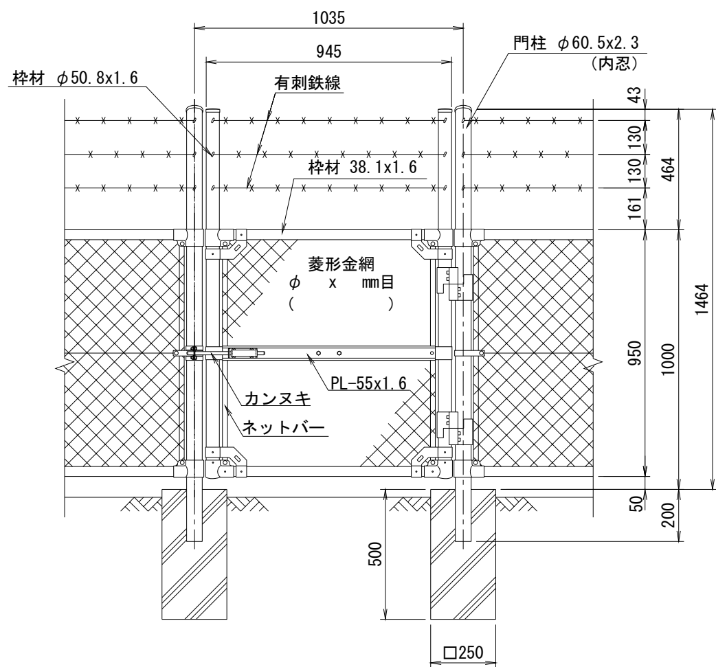
正面図 (S=1/20)
