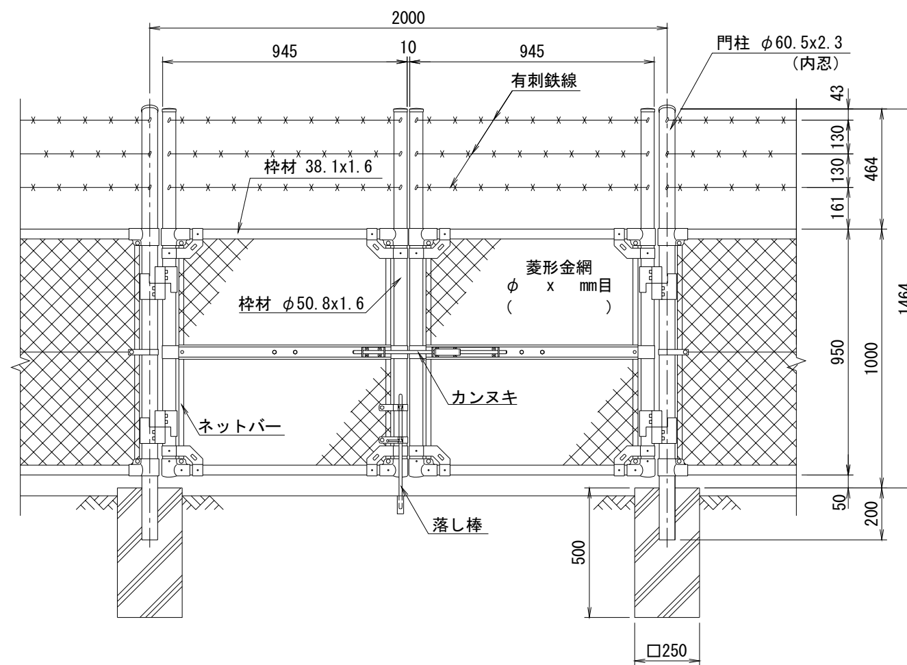
正面図 (S=1/20)
