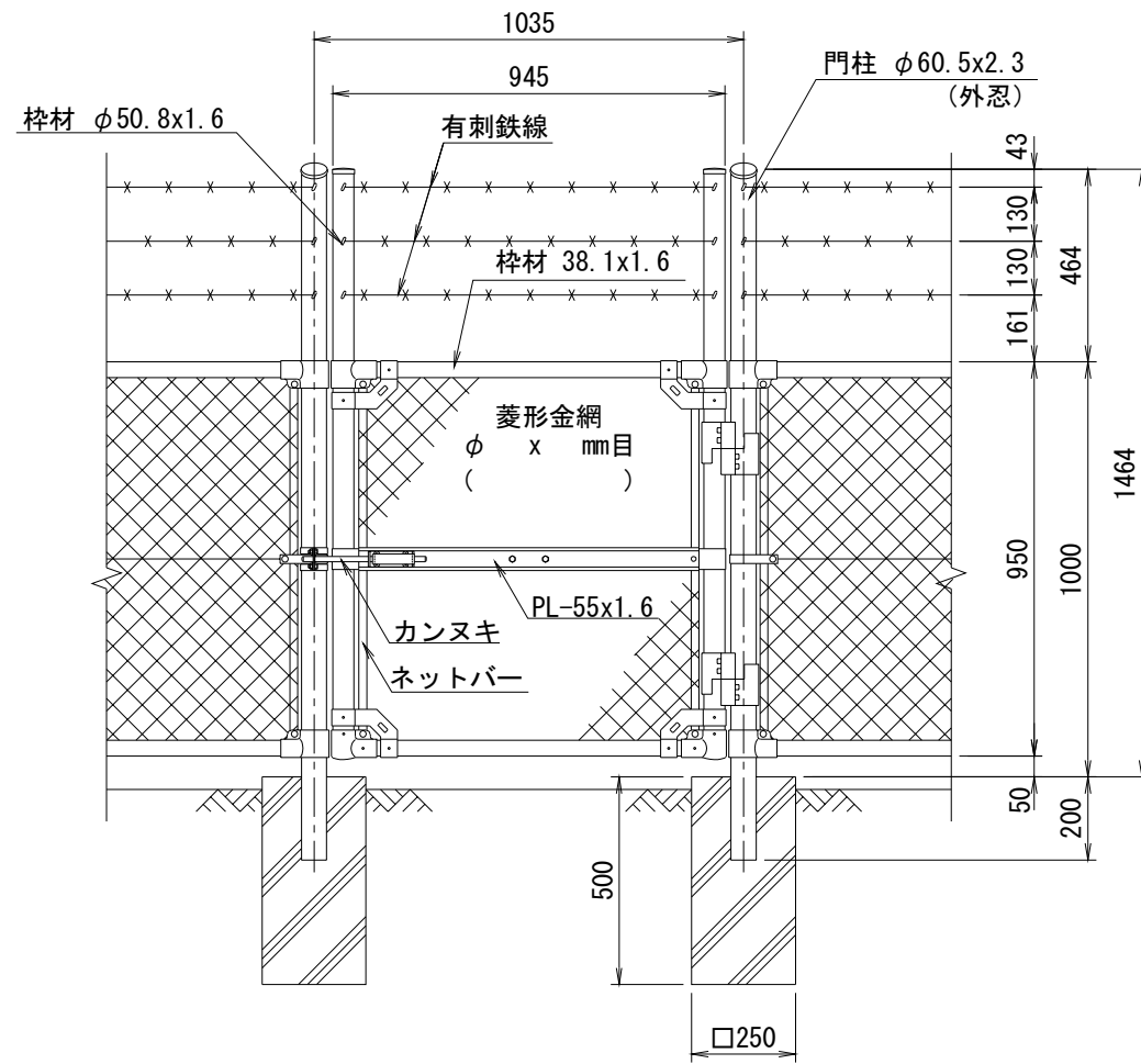
正面図 (S=1/20)
