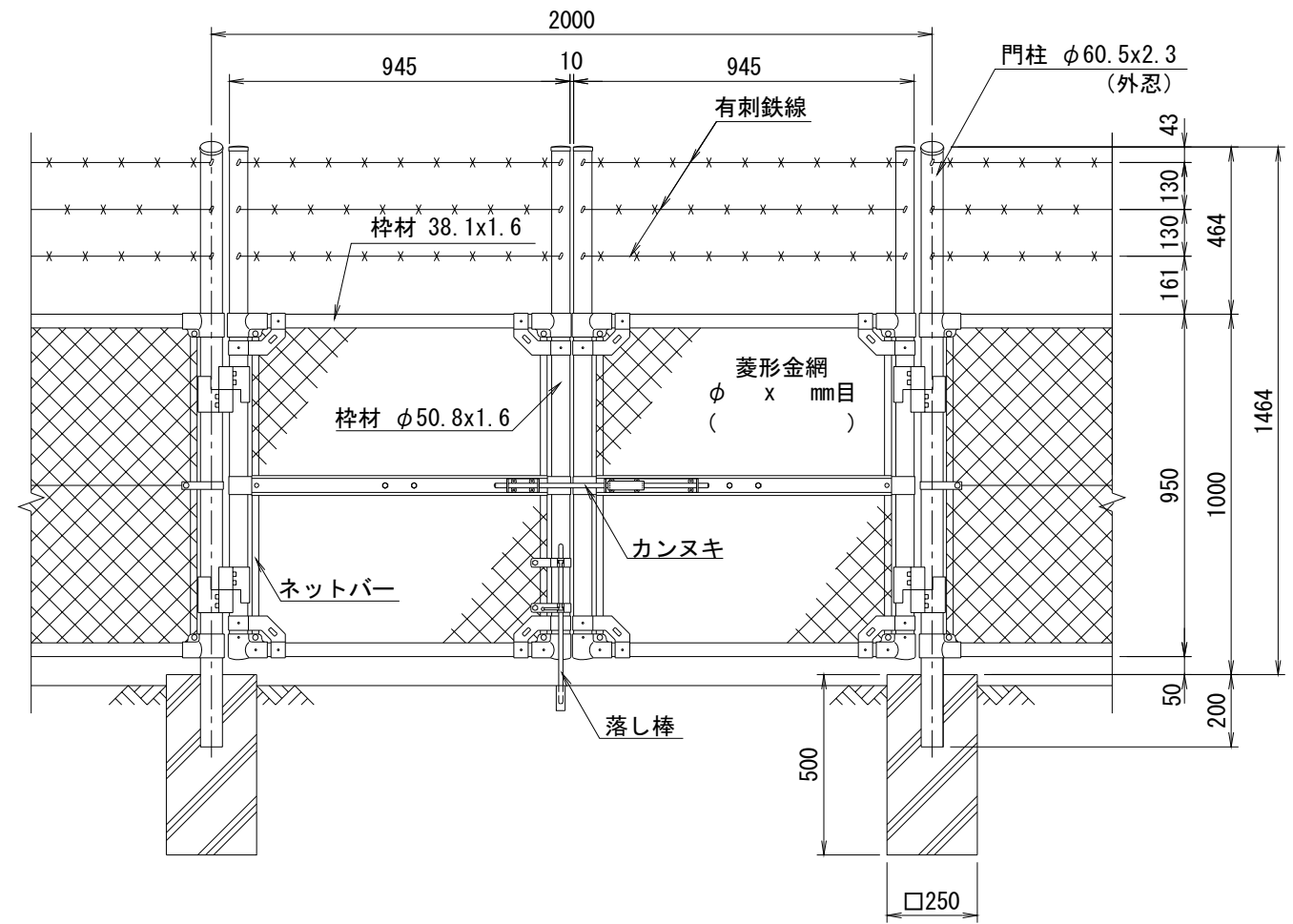
正面図 (S=1/20)
