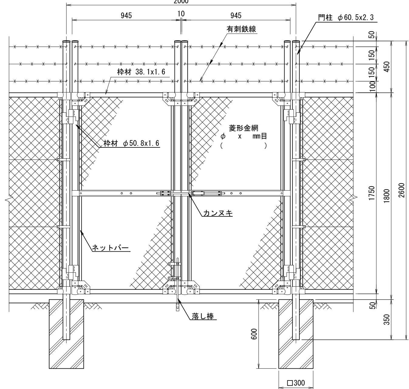
正面図
