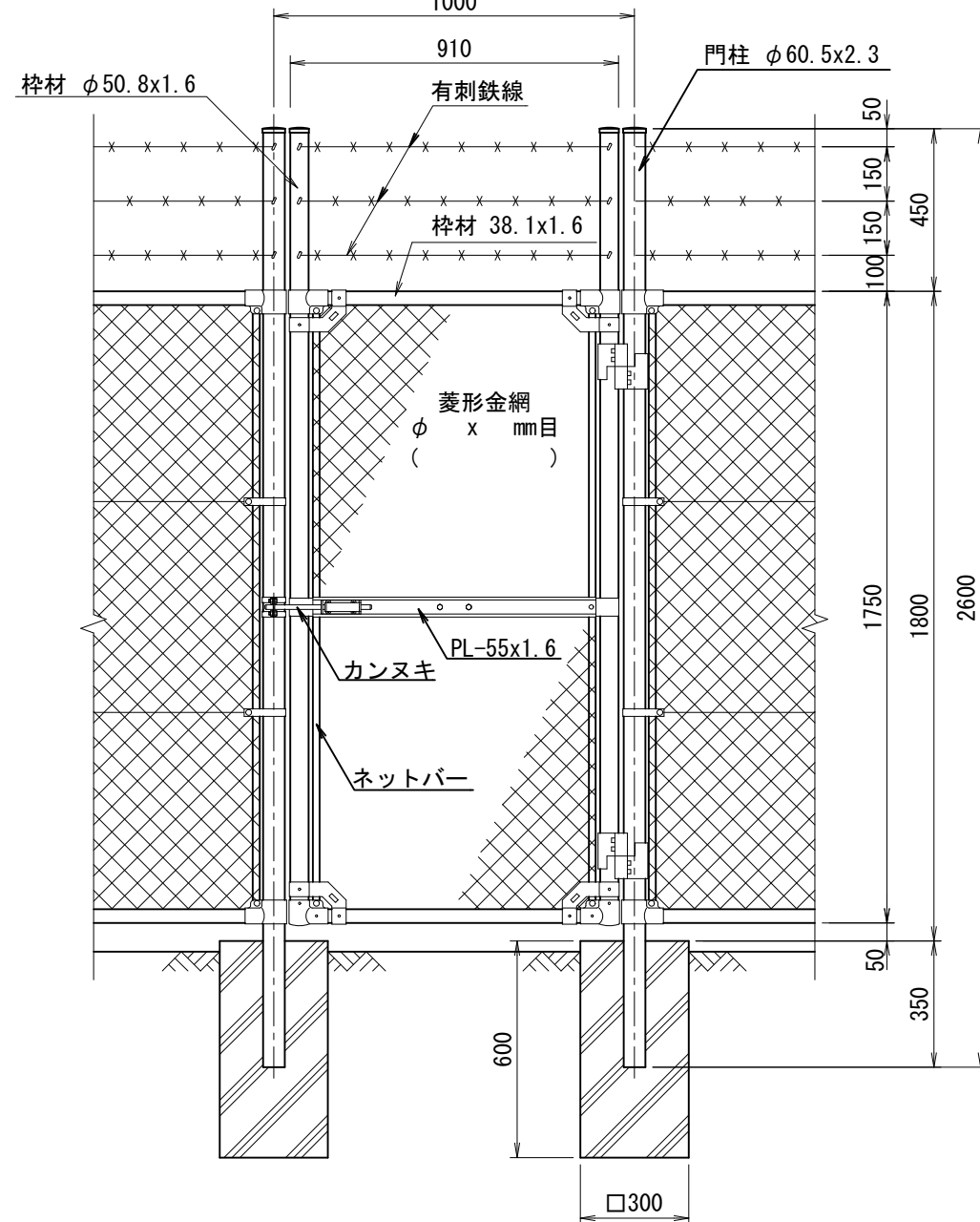
正面図
