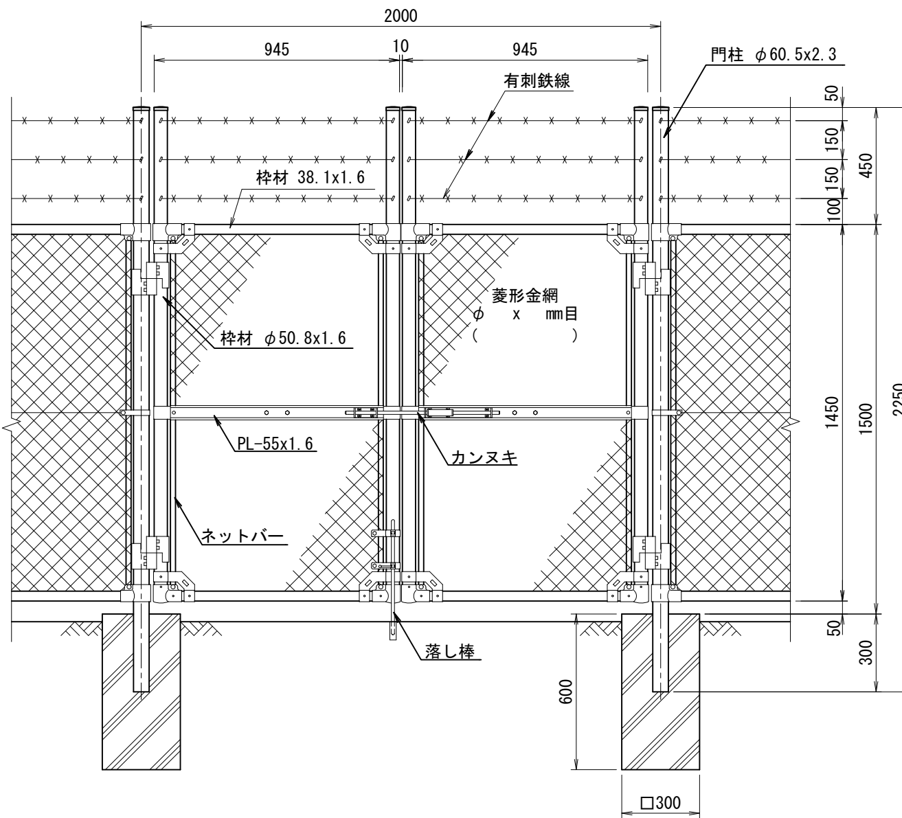
正面図 (S=1/20)
