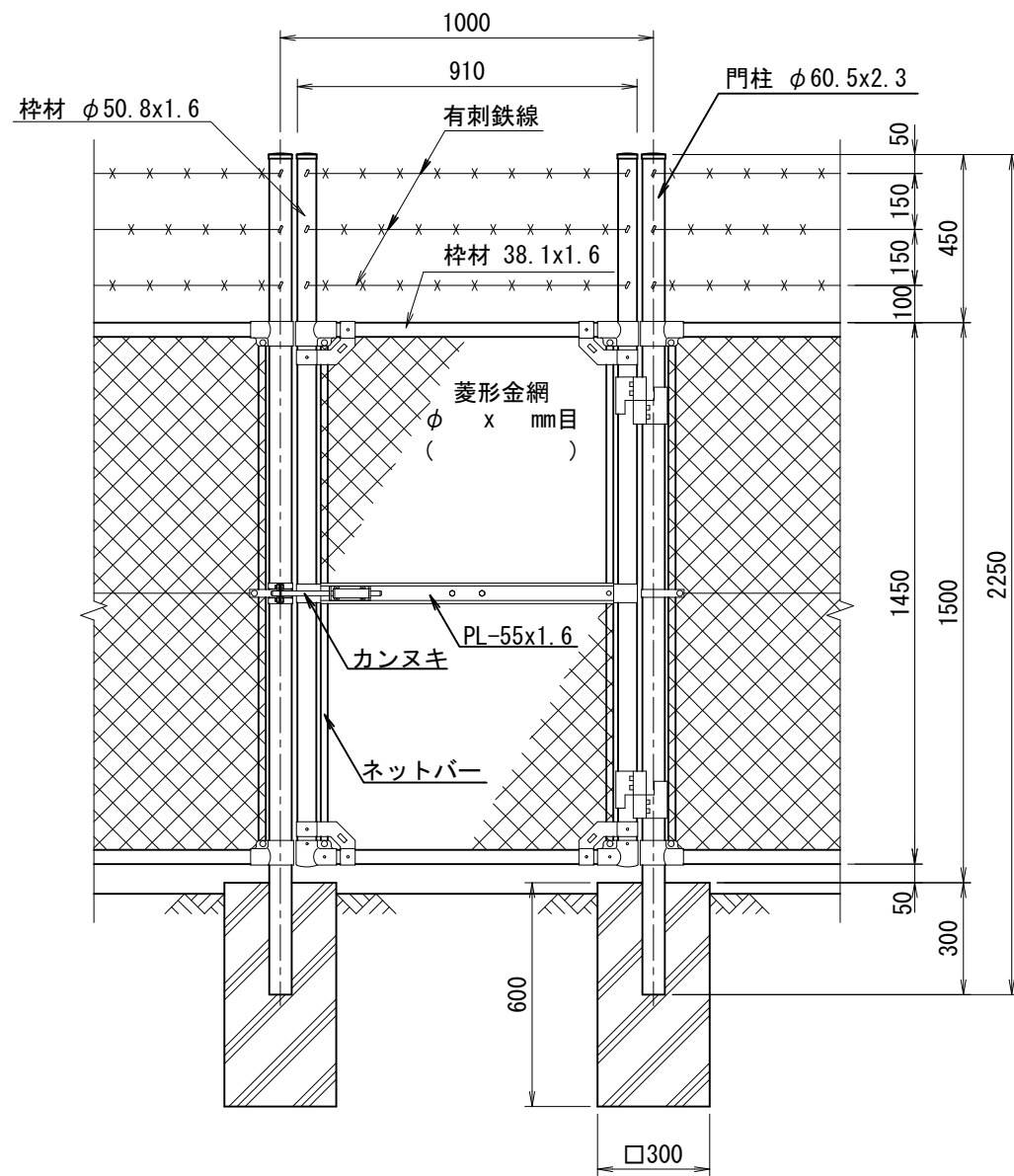
正面図 (S=1/20)
