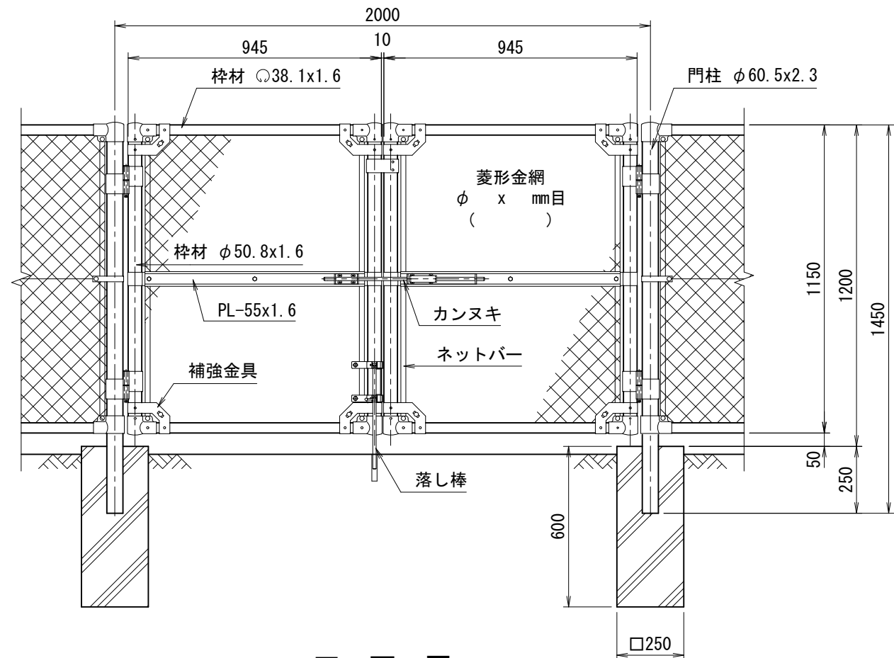
正面図 (S=1/20)
