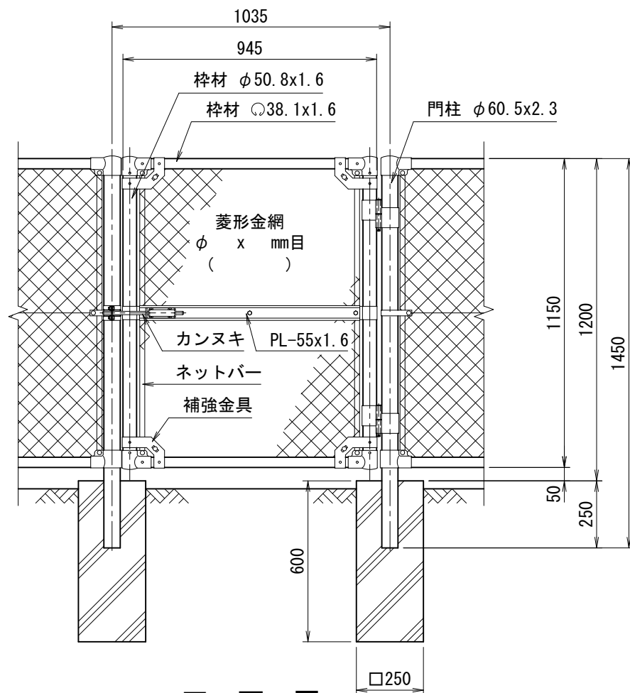
正面図 (S=1/20)
