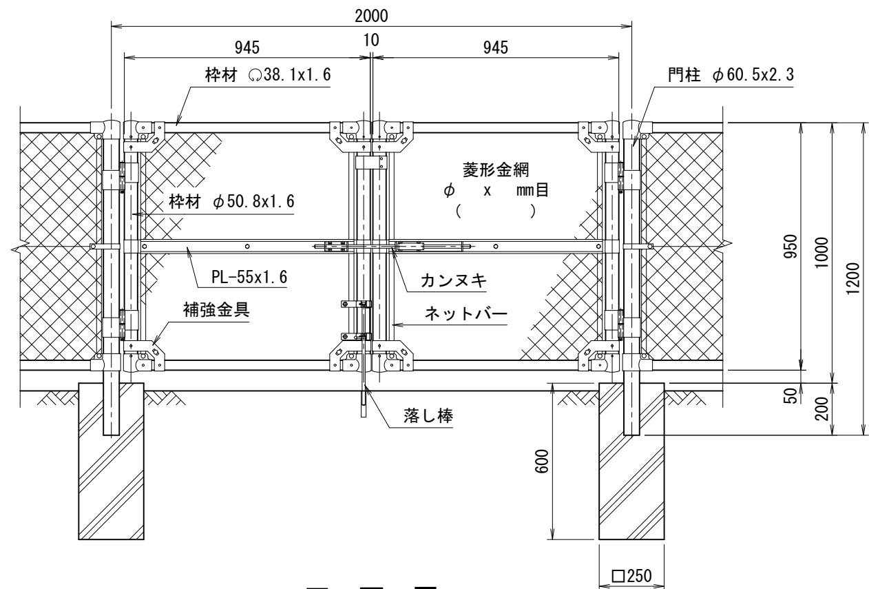
正面図 (S=1/20)
