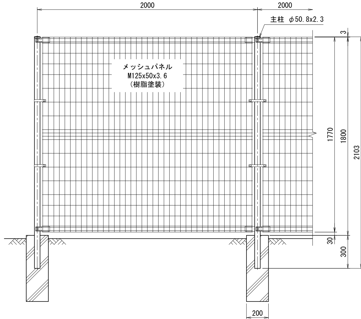
正面図 (S=1/20)
