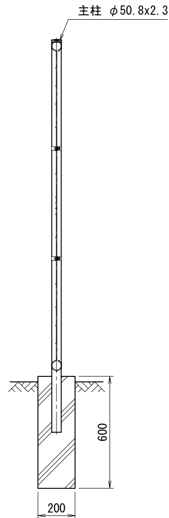
側面図 (S=1/20)
